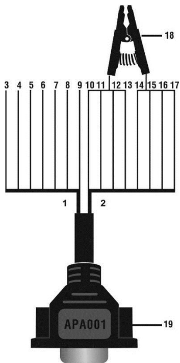
图 2-5 EEPROM 夹具集成 MC9S12 线束
