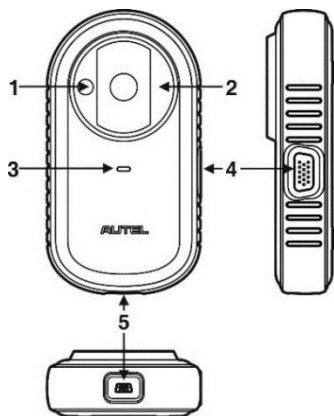
图 2-4 专用编程器 XP201 图示
