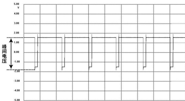
图 16-2 方波示图
