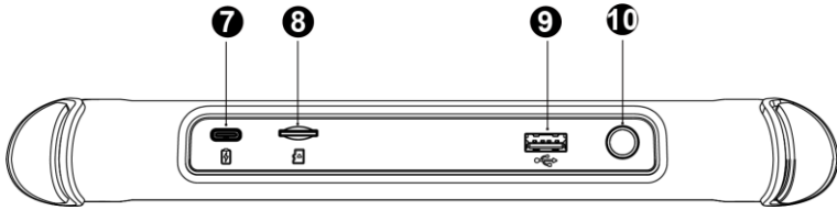
图 2-3 MS906S2-BT 平板诊断设备顶视图
