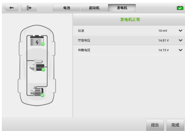
图 11-8 “发电机检测结果” 界面示图
